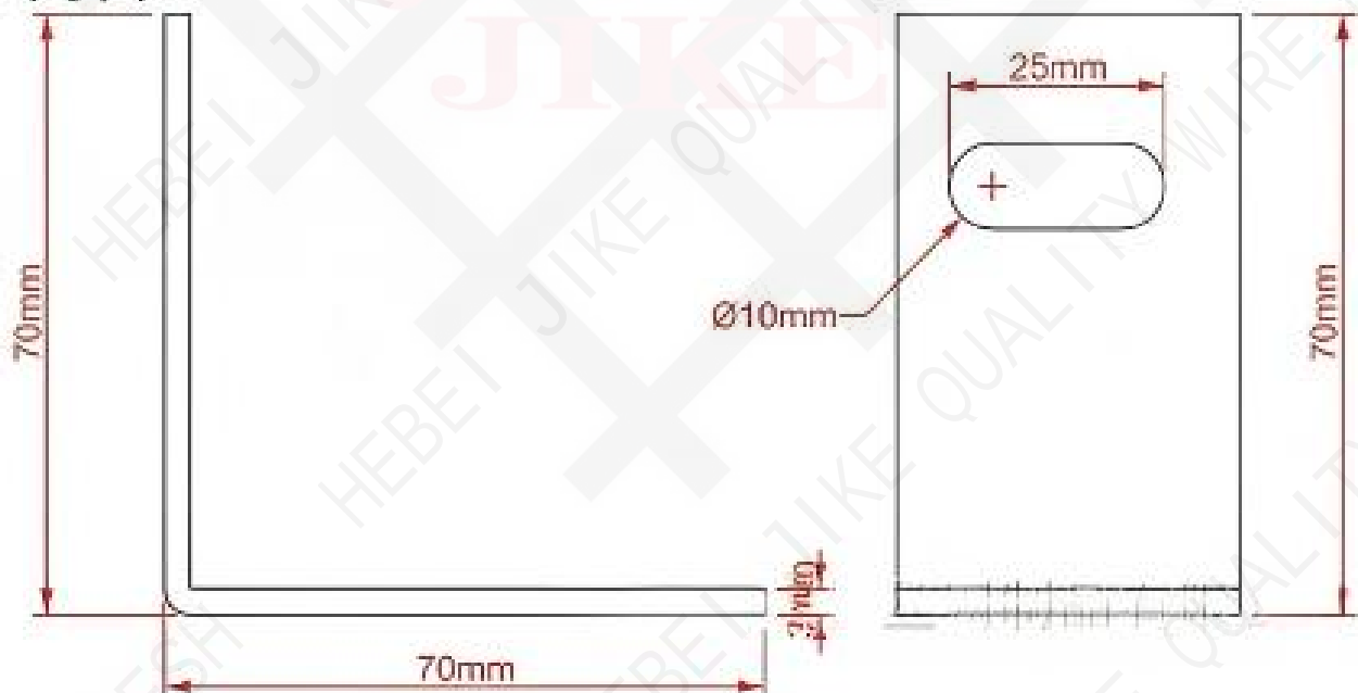
产品尺寸图：
