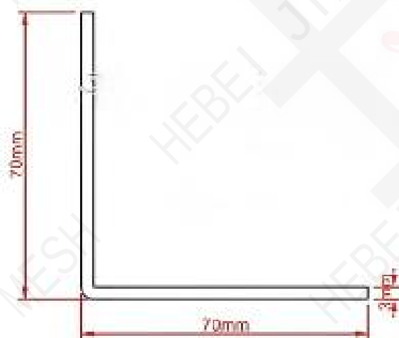
产品尺寸图：
