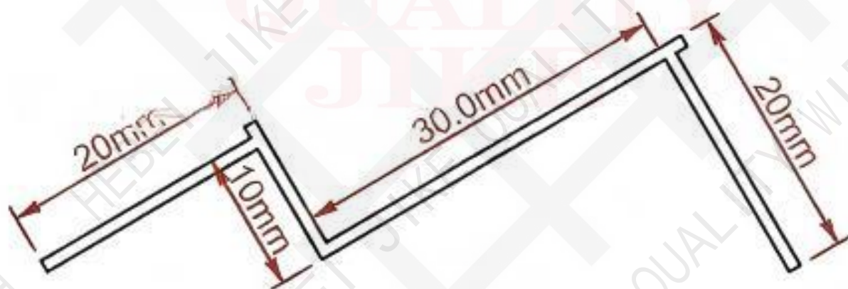
产品尺寸图:
