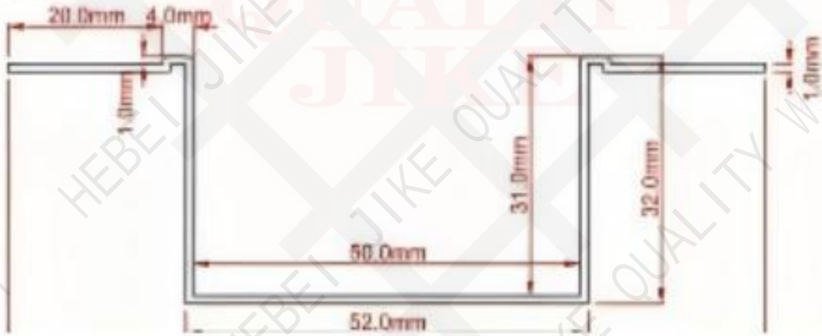
产品尺寸图：
