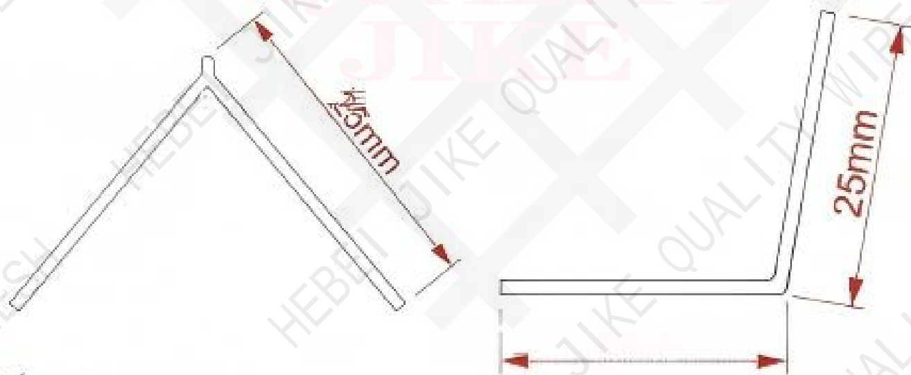
产品尺寸图：
