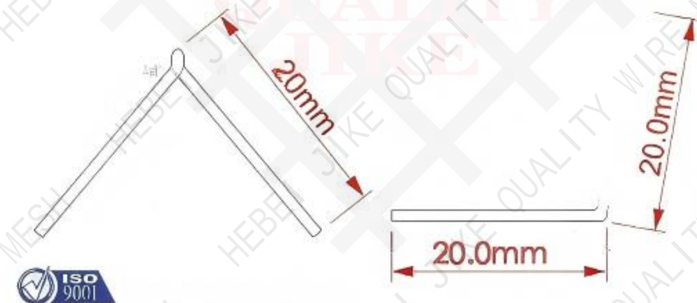
产品尺寸图：
