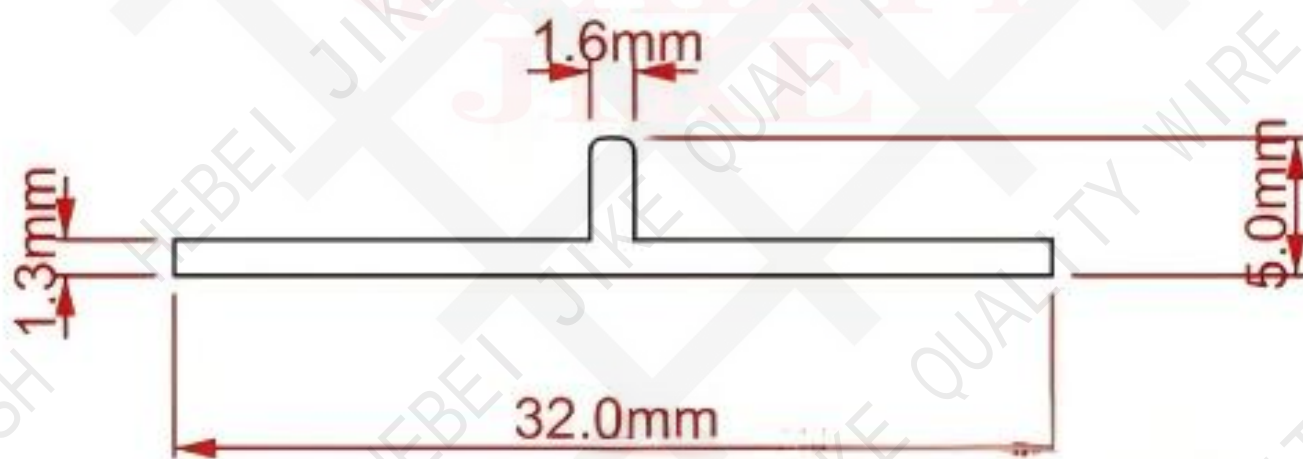
产品尺寸图：
